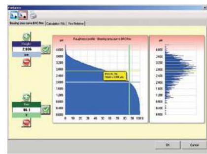
Curva di portanza
