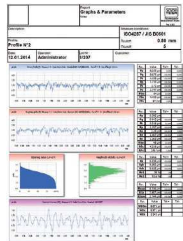
Report di misura con intestazione e logo personalizzabili
