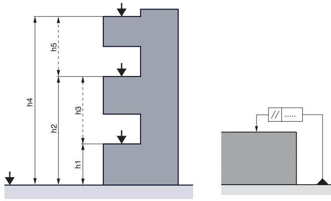
Misure in una direzione di coordinata
