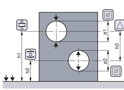
Misure con inversione del senso di tastatura Con costante di tastatura, con memorizzazione del punto di inversione
