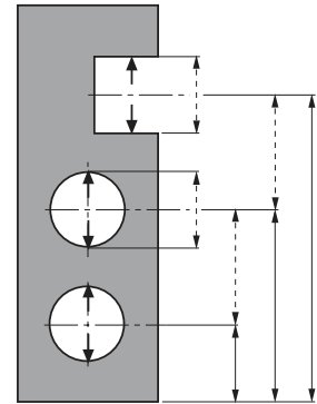
Misure in una direzione di coordinata
