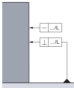
Rilevamento di errori di forma e posizione
